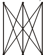
K_{3,3}
